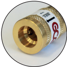
Schnellkupplung nach EN561 / ISO 7289
