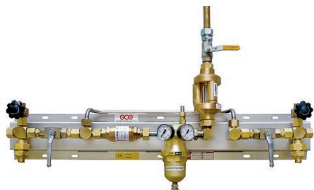
Acetylen-Versorgung
